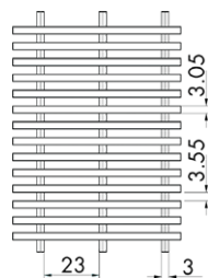
Tile Insert
