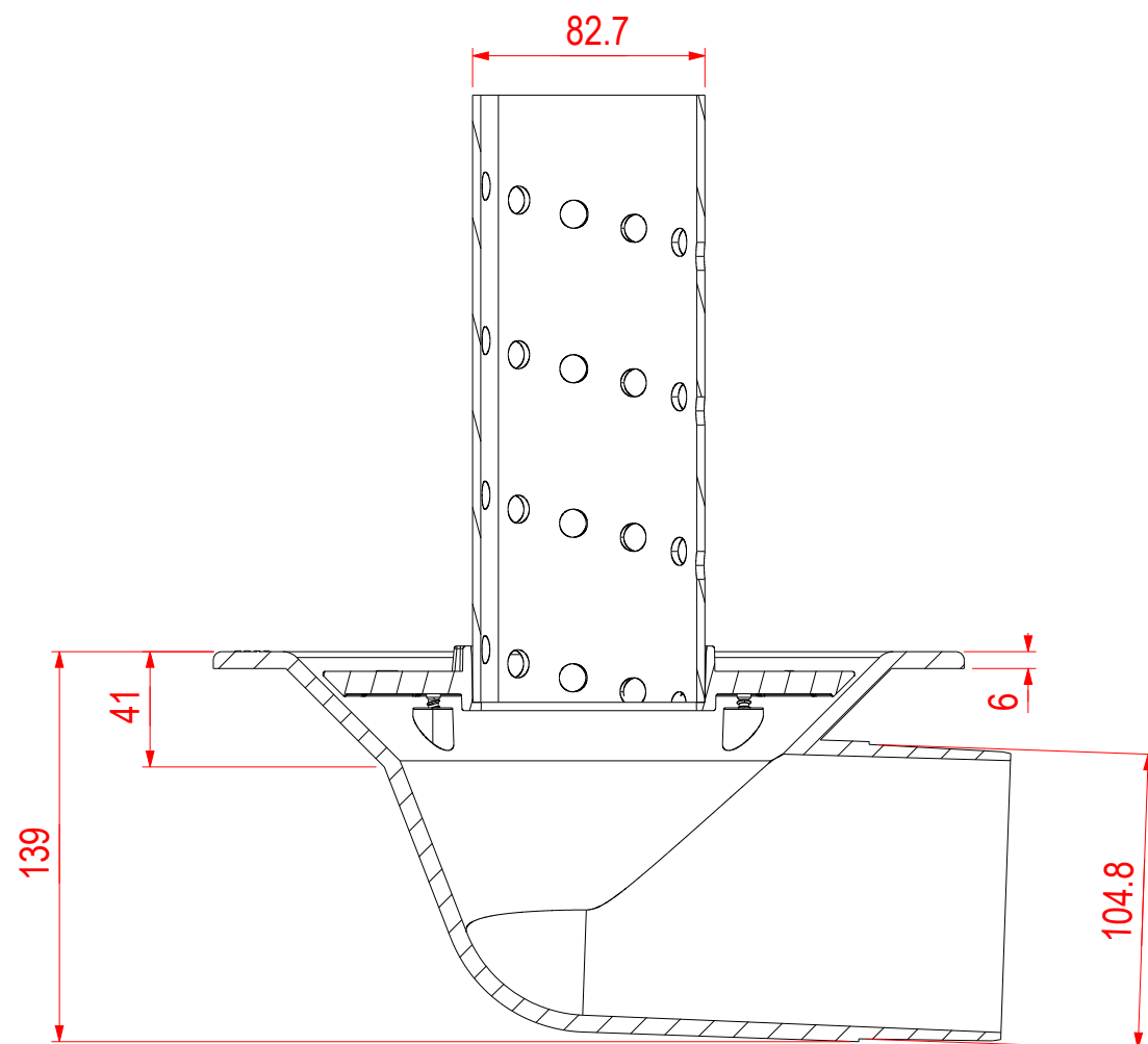
Section A-A
